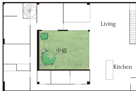
2F Plan 中庭は6.5 m×5.3 mの広さ
