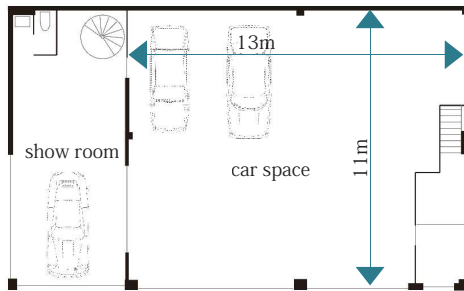
1F Plan Car spaceは13 m×11 mの大空間です。
